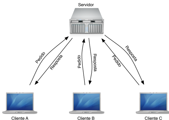
Figura 3.1: Modelo Cliente-Servidor
