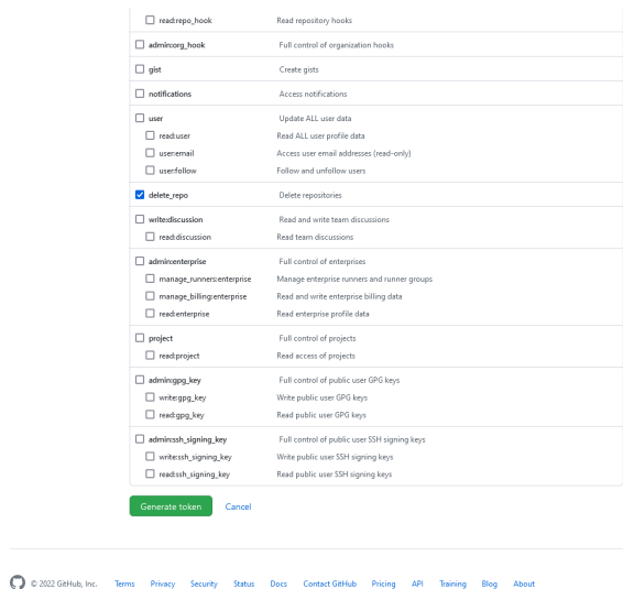
Figura 4.15: Parte inferior da página de requisição do token de segurança.
